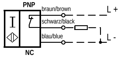
3RG4012-0AF33-PF:
