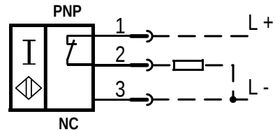
3RG4012-3AF33-PF:
