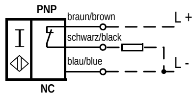
3RG4022-0AF30-PF:
