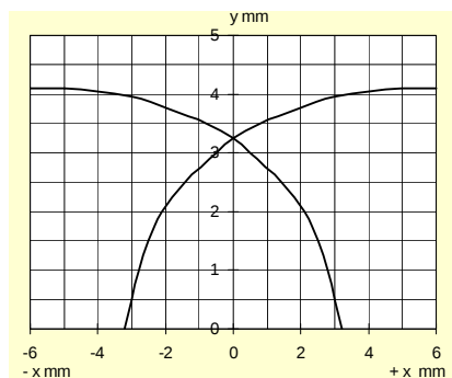
Response characteristics/Ansprechkennlinie:
