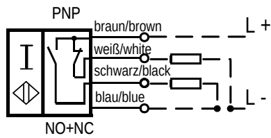
3RG4023-0CD00-PF:
