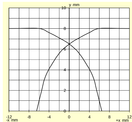
Response characteristics/Ansprechkennlinie:
