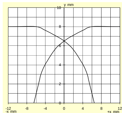
Response characteristics/Ansprechkennlinie:
