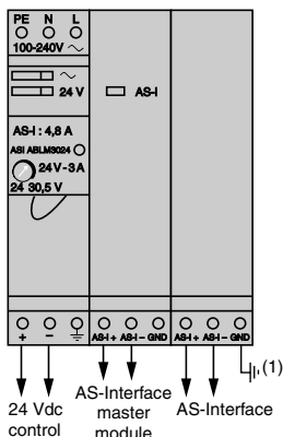
ASIABLM3024
