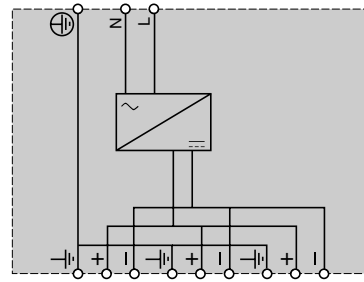
ABL7RE2410
