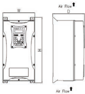
Frame 1 (IP66)
