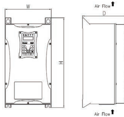
Frame 3 (IP66)
