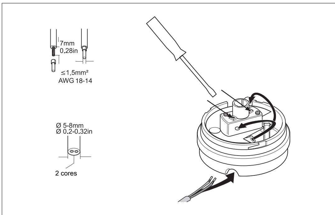
Fig.: Wiring
